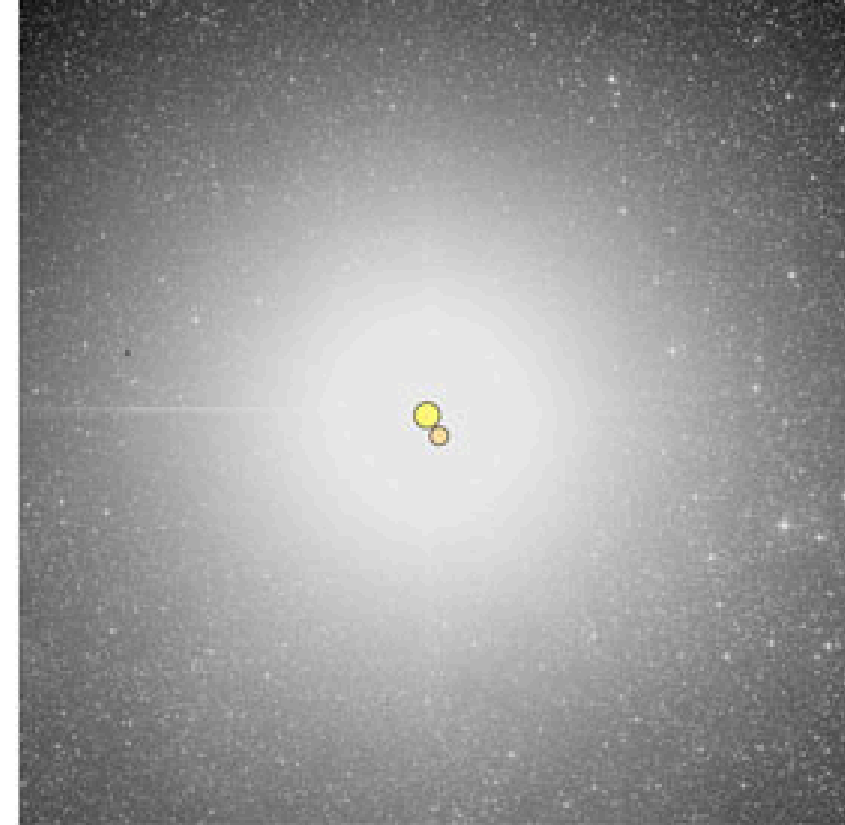
\alpha Cen A & B
